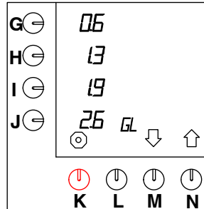
Fig. 29 Endring av forhåndsprogrammerte valgtaster for gallons
