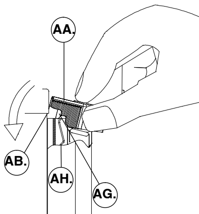
Fig. 9 Plassering og avtaking av glassdekslet
